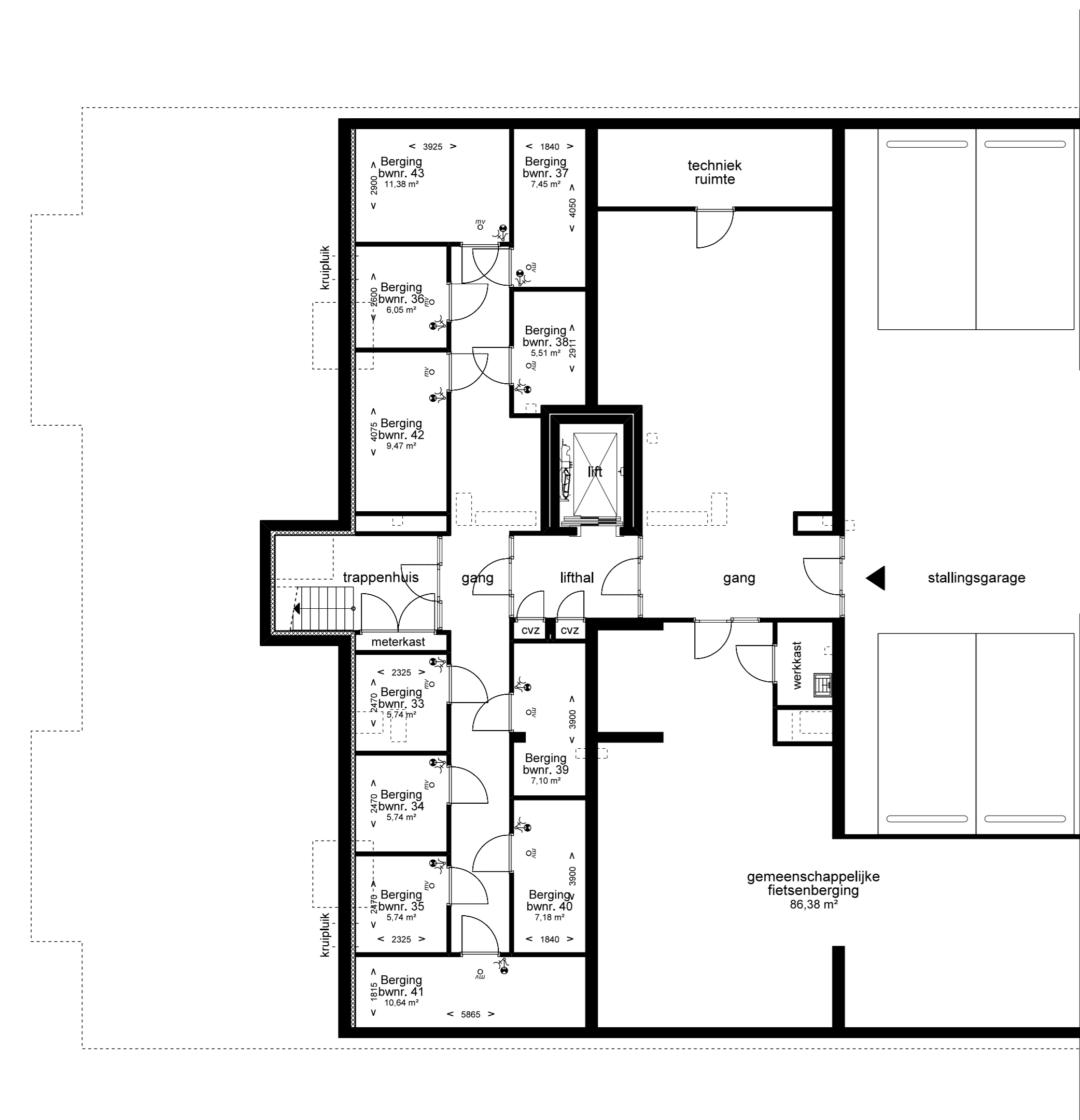
KELDER
