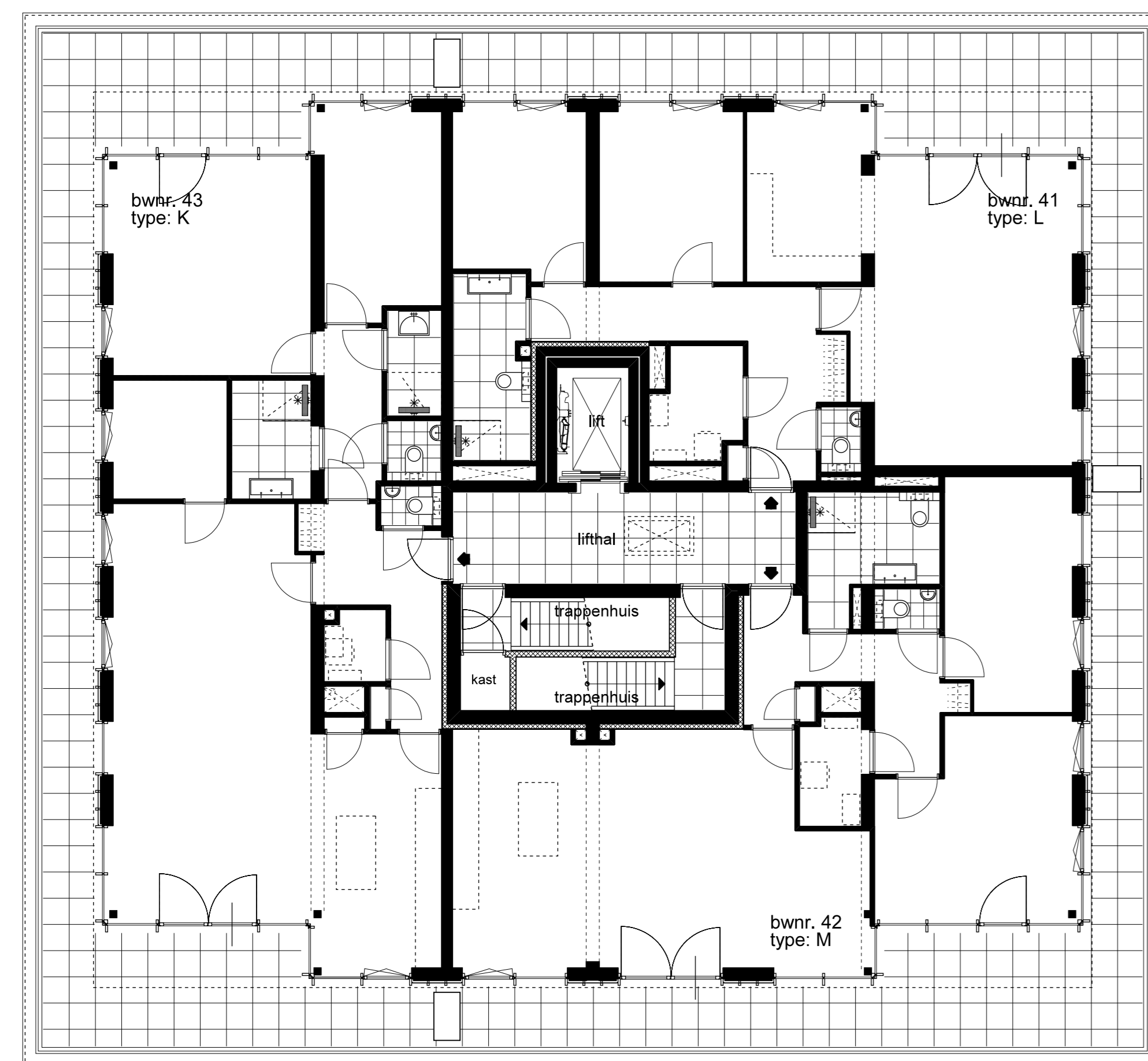
2e VERDIEPING
