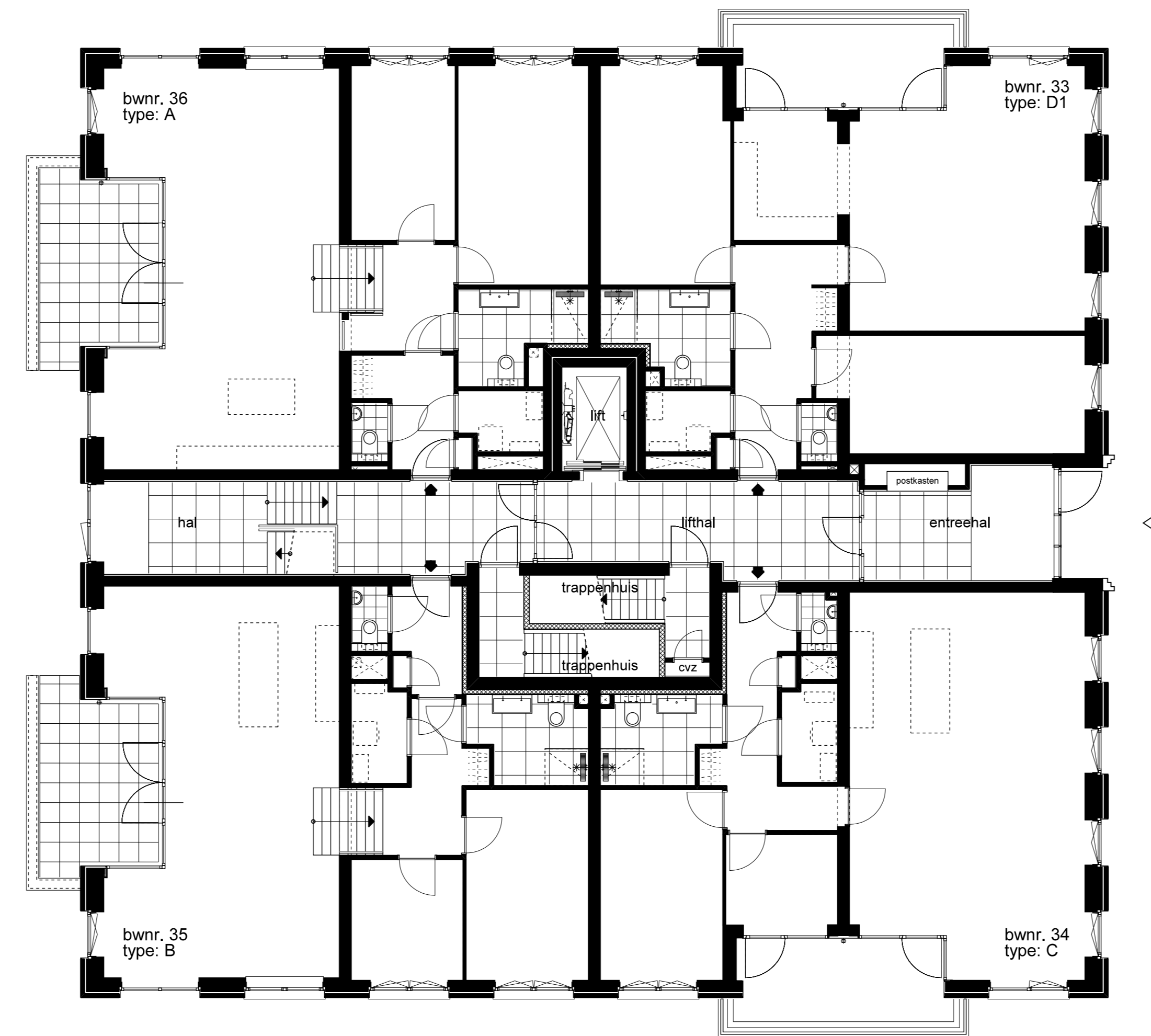
BEGANE GROND
